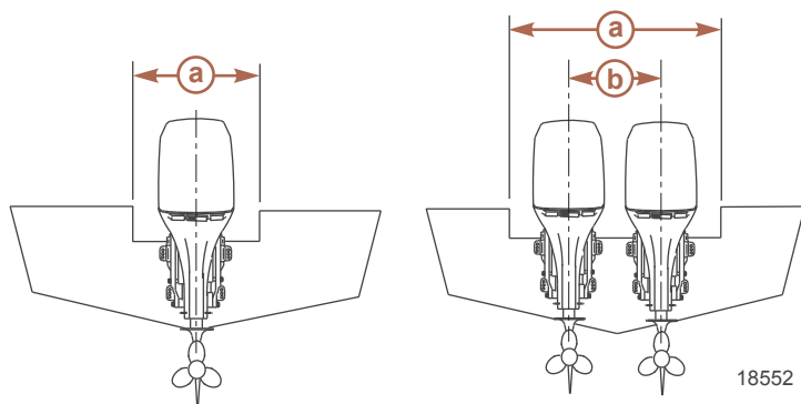
a - Minimálny otvor pričky
